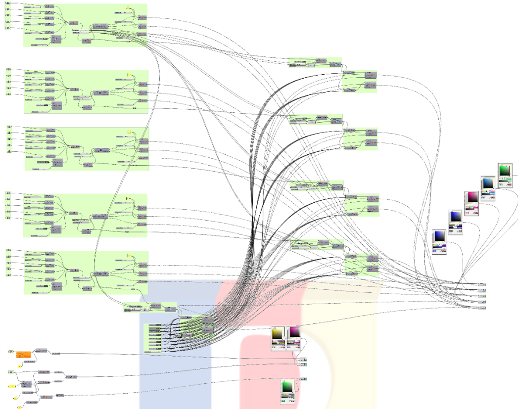
Rumus Simulasi Membrane Roof (Kangaroo 2) & Truss System pada Peron AKDP
