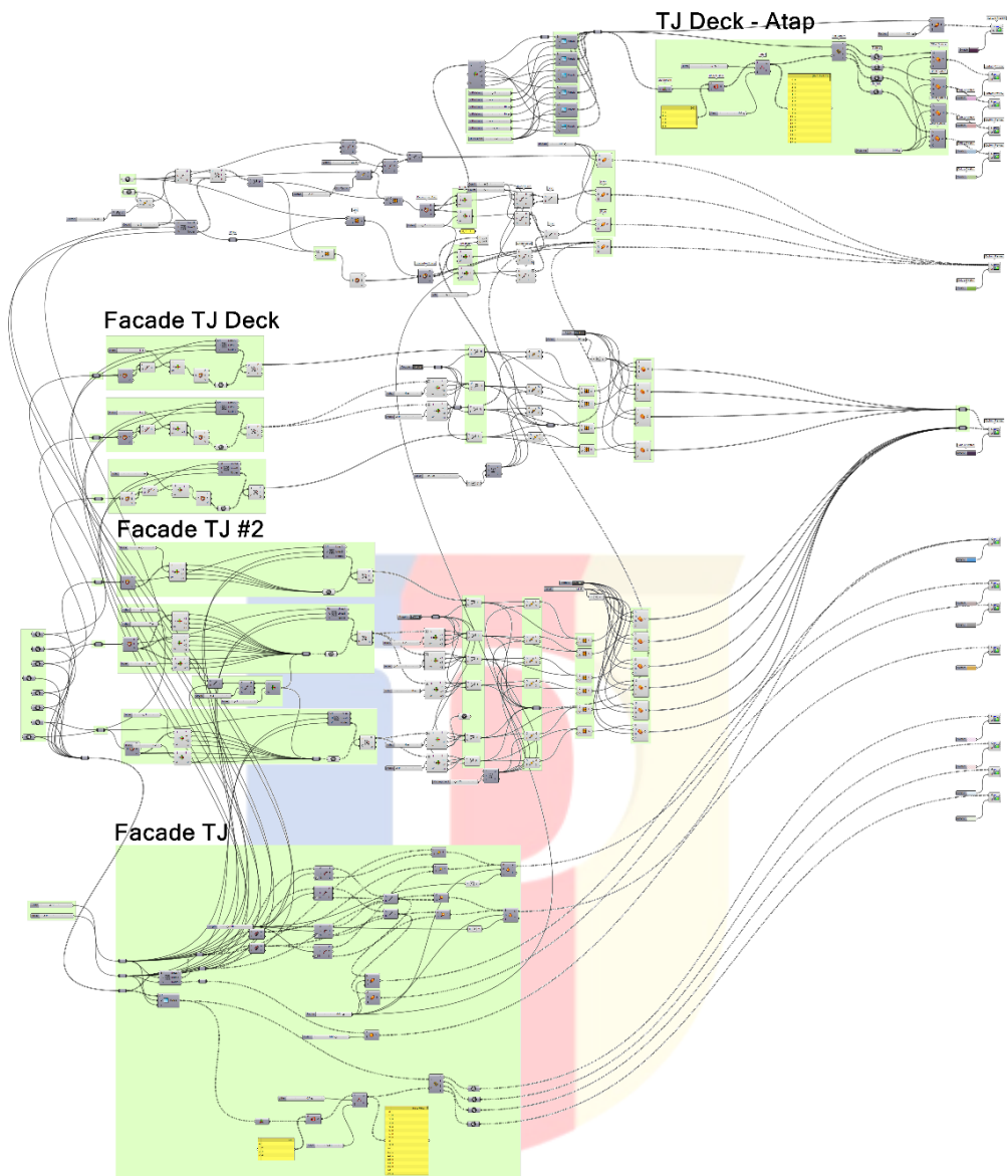
Rumus Simulasi Facade Truss System pada Halte TransJakarta
