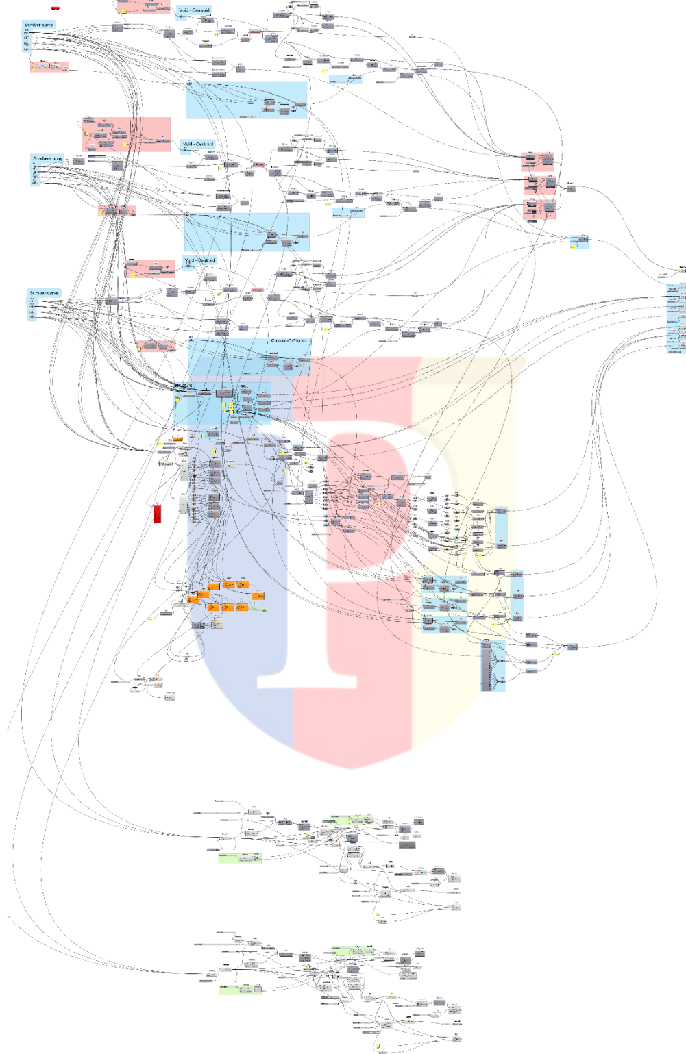
Rumus Simulasi Membrane Roof (Kangaroo 2) & Truss System pada Peron TransJakarta
