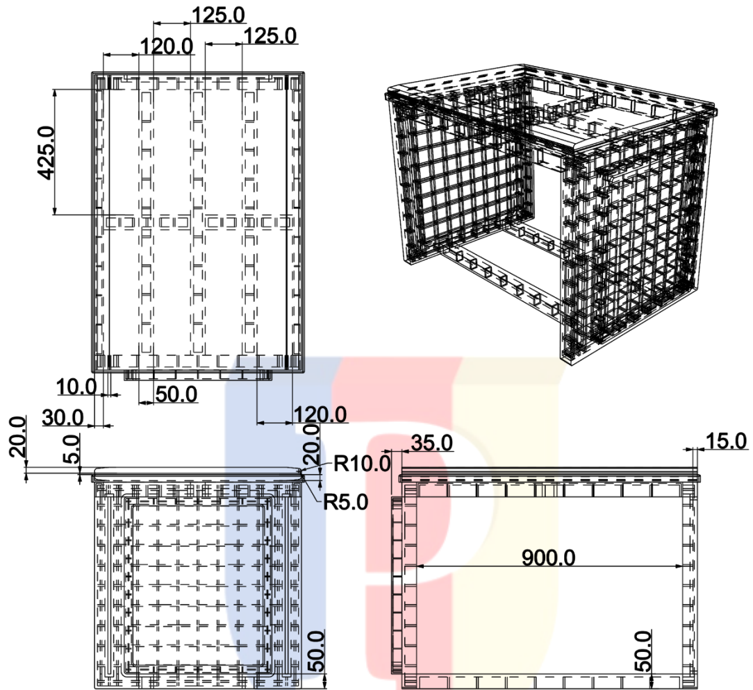
Lampiran 7 Gambar Teknik Detail Modul Utama
