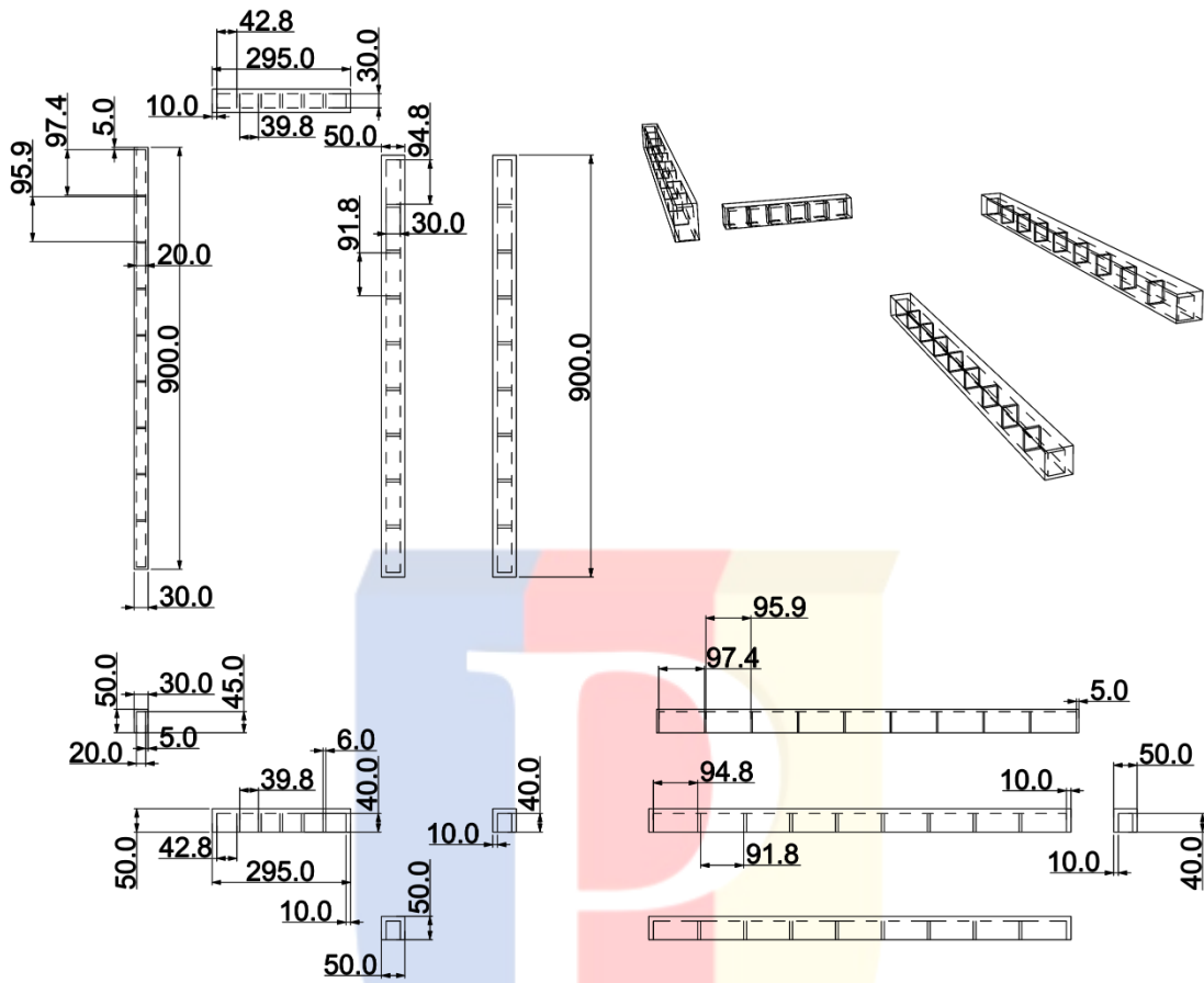
Lampiran 12 Gambar Teknik Ribbing Modul Utama Bagian Penyangga
