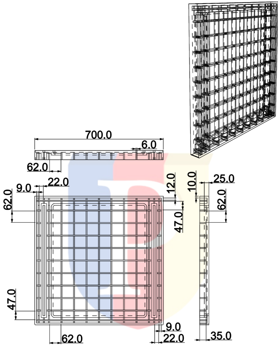
Lampiran 10 Gambar Teknik Ribbing Modul Utama Bagian Samping
