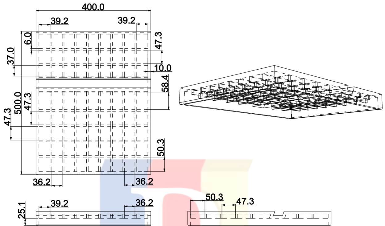
Lampiran 19 Gambar Teknik Ribbing Modul Kursi Dasar
