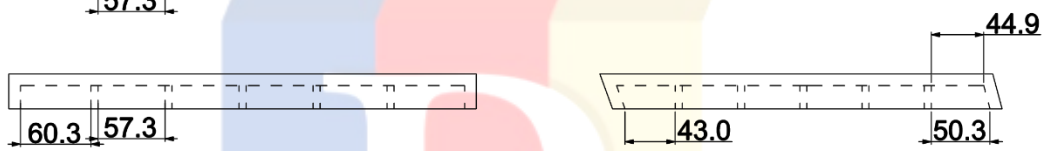
Lampiran 23 Gambar Teknik Ribbing Modul Kursi Bagian Sekat
