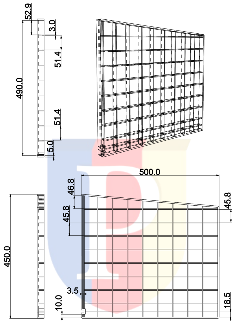
Lampiran 18 Gambar Teknik Ribbing Modul Kursi Bagian Samping
