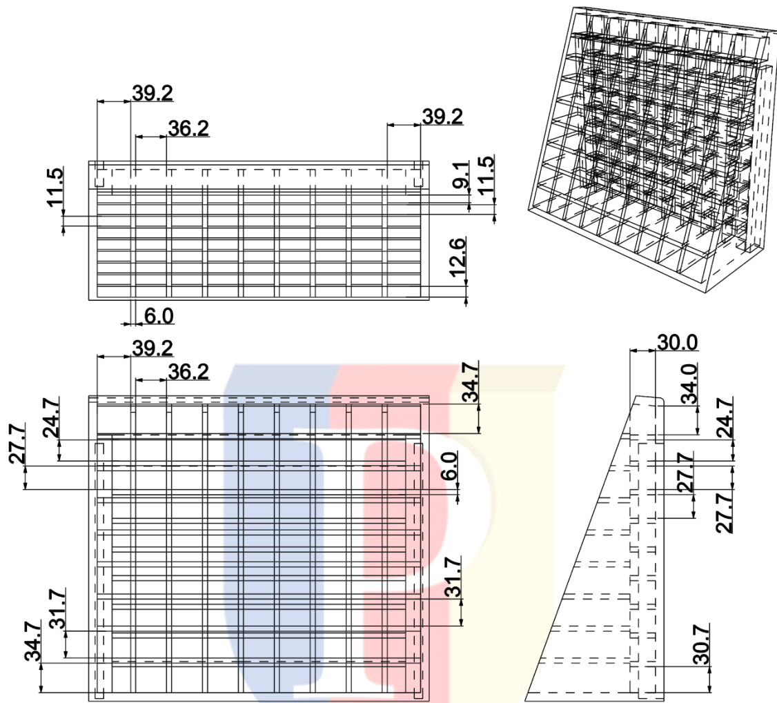
Lampiran 21 Gambar Teknik Ribbing Modul Kursi Bagian Belakang
