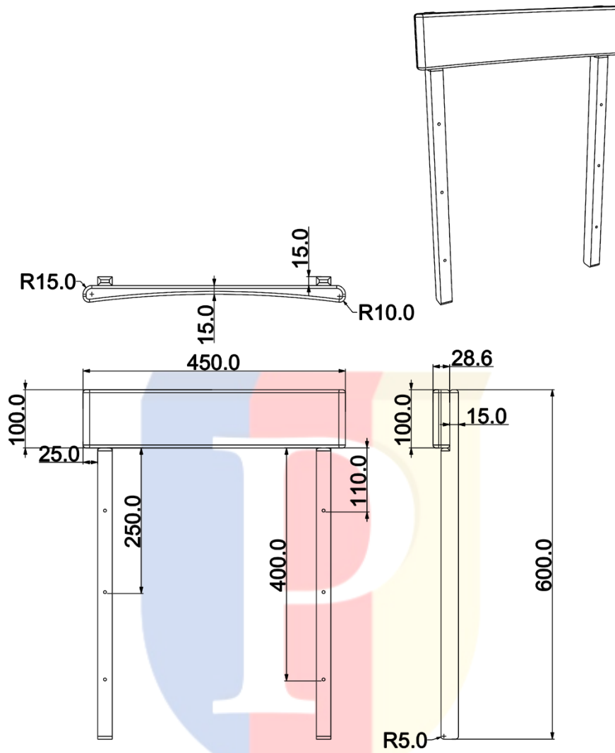
Lampiran 22 Gambar Teknik Ribbing Modul Kursi Bagian Sandaran
