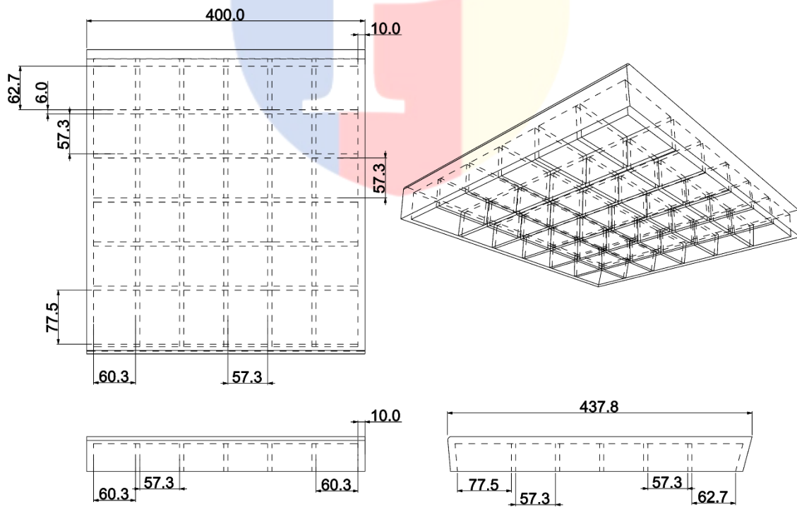
Lampiran 20 Gambar Teknik Ribbing Modul Kursi Bagian Dudukan
