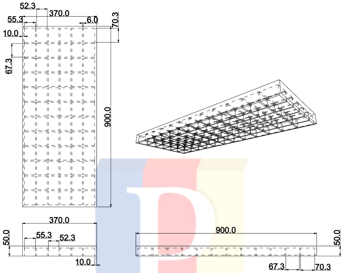
Lampiran 15 Gambar Teknik Ribbing Modul Tambahan Bagian Dasar
