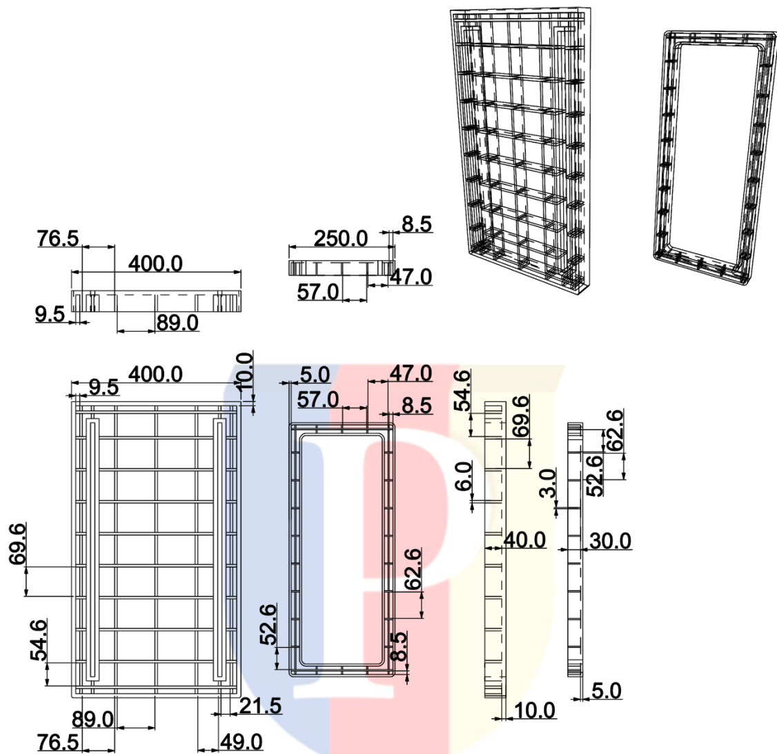
Lampiran 14 Gambar Teknik Ribbing Modul Tambahan Bagian Samping 2
