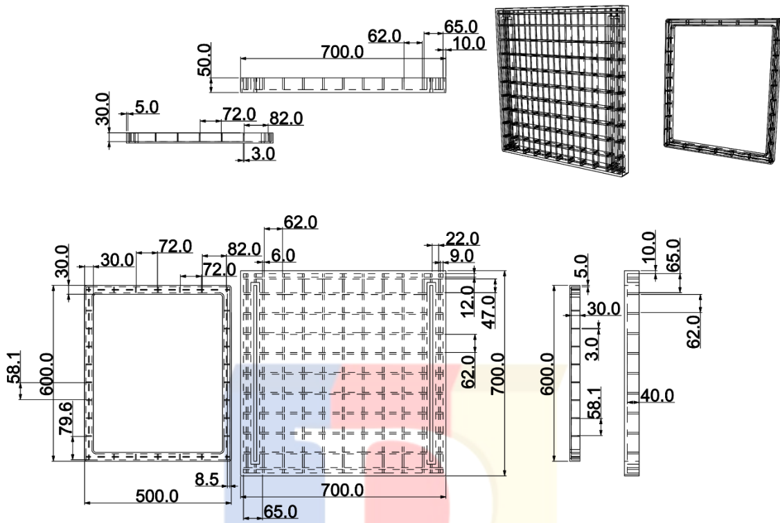
Lampiran 11 Gambar Teknik Ribbing Modul Utama Bagian Samping 2
