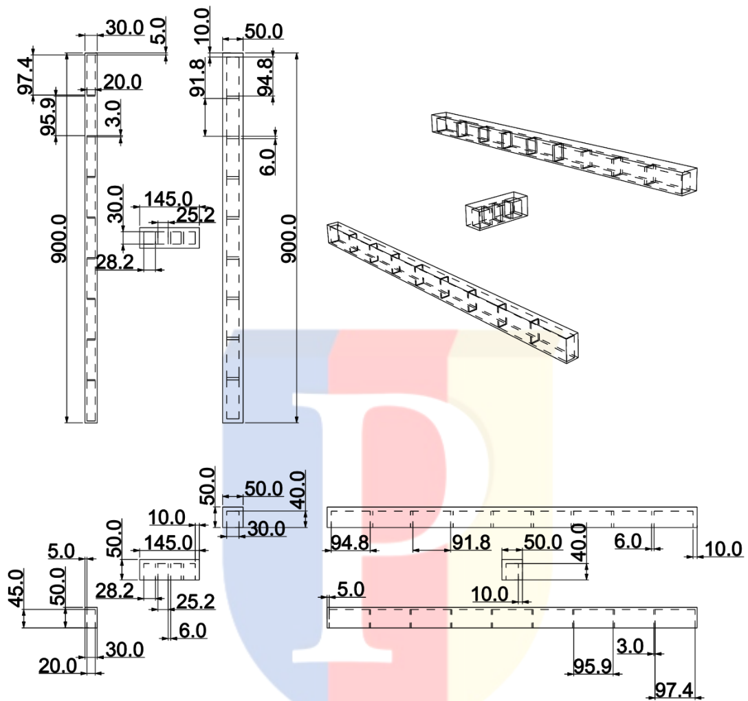
Lampiran 17 Gambar Teknik Ribbing Modul Tambahan Bagian Penyangga
