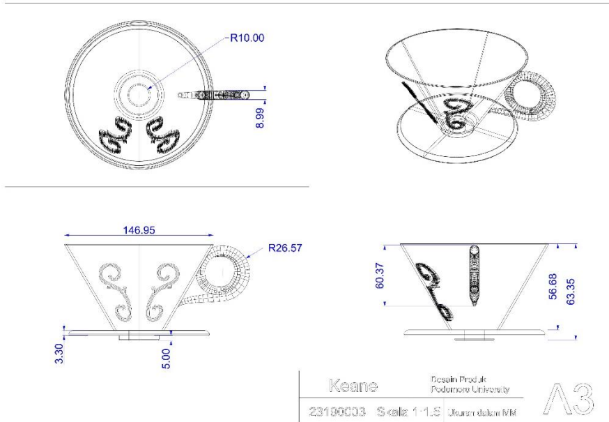
Gambar 5.8 Gambar Teknik
