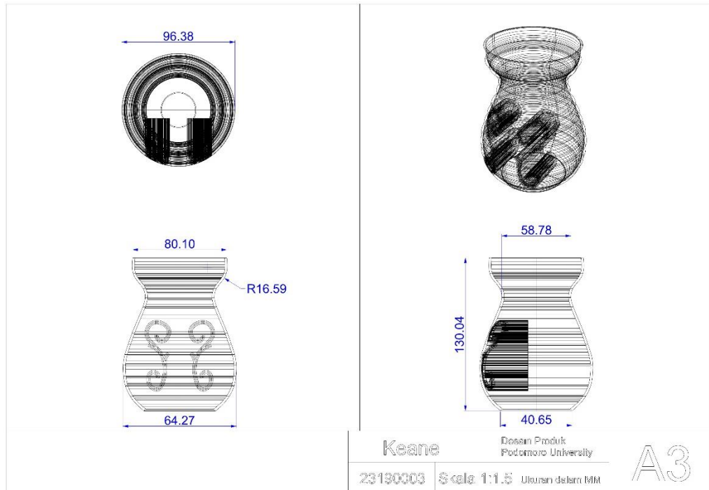
Gambar 5.10 Gambar Teknik
